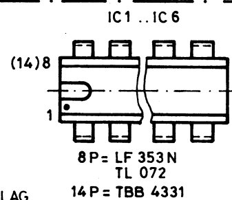
VON OBEN GESEHEN TOP VIEW
