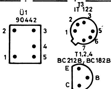
AUF DIE STIFTE GESEHEN PIN VIEW
