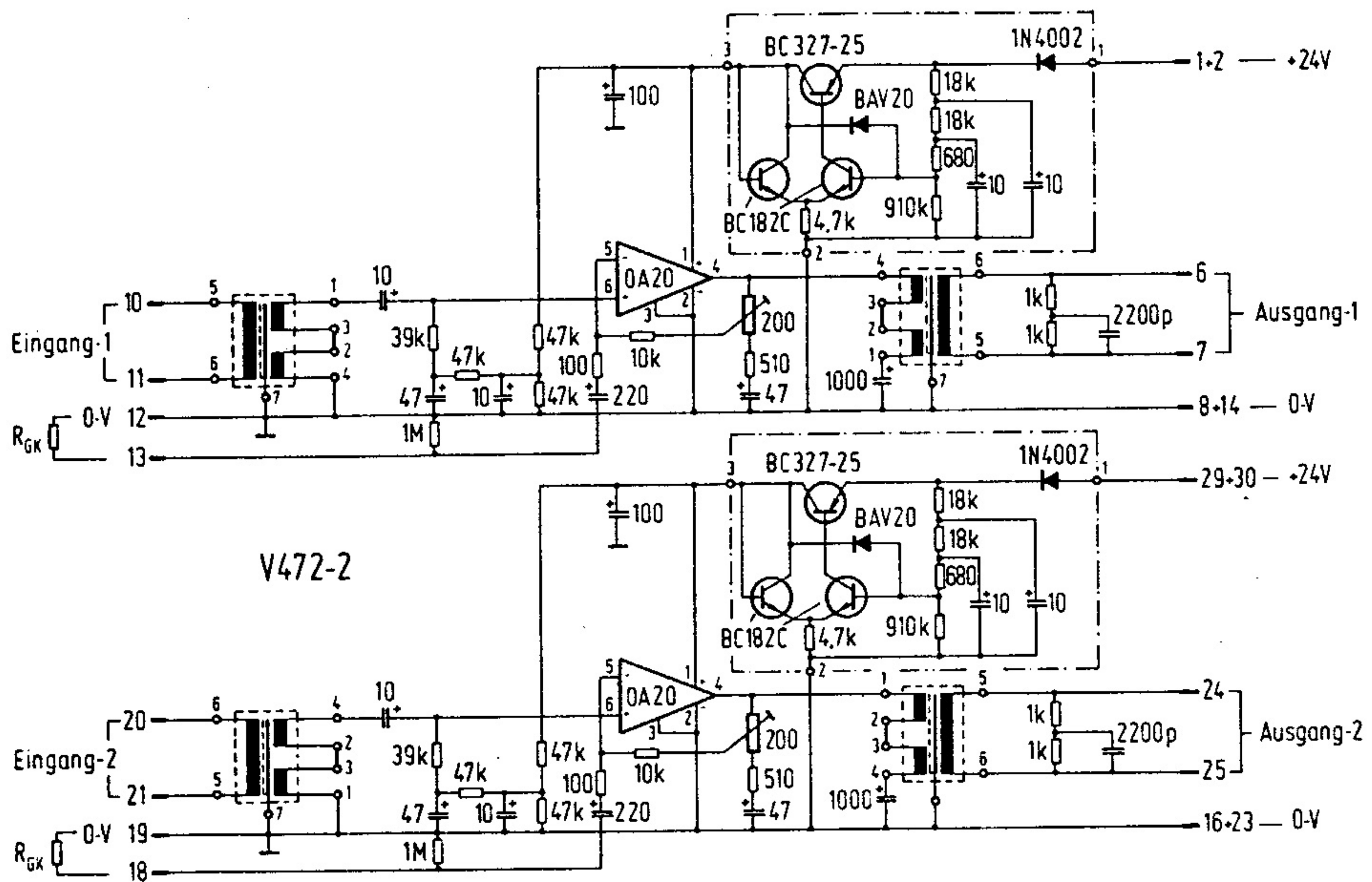
Bild E 65. Ausgangs- und Trennverstärker V472-2 (Neumann)
