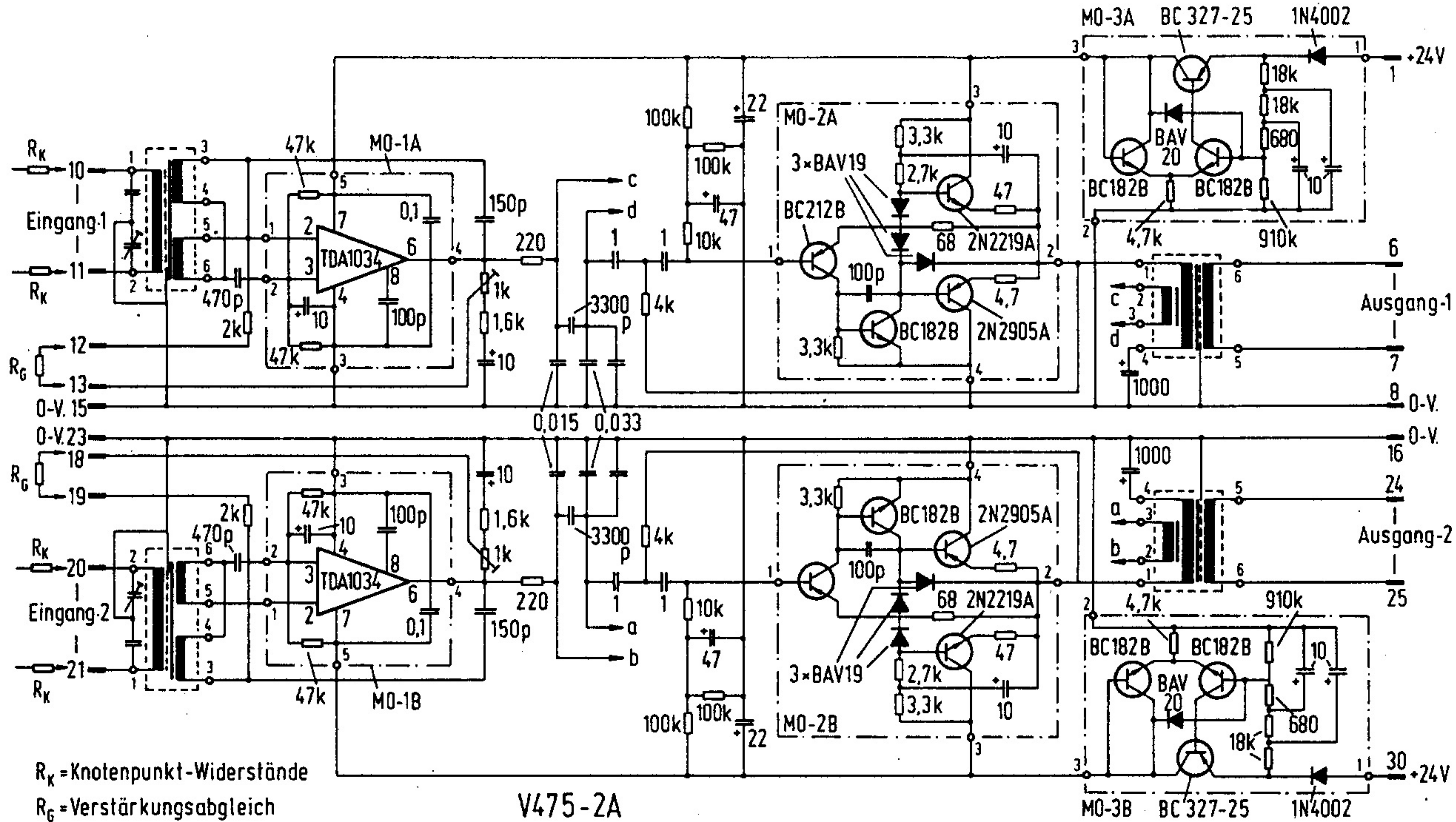
Bild E 63. Doppel-Knotenpunktverstärker V 475 (Neumann). Die einzelnen Ausgänge der Mikrofonkanäle werden über die Entkopplungswiderstände R_K am jeweiligen Knotenpunkteingang zusammengefaßt.
