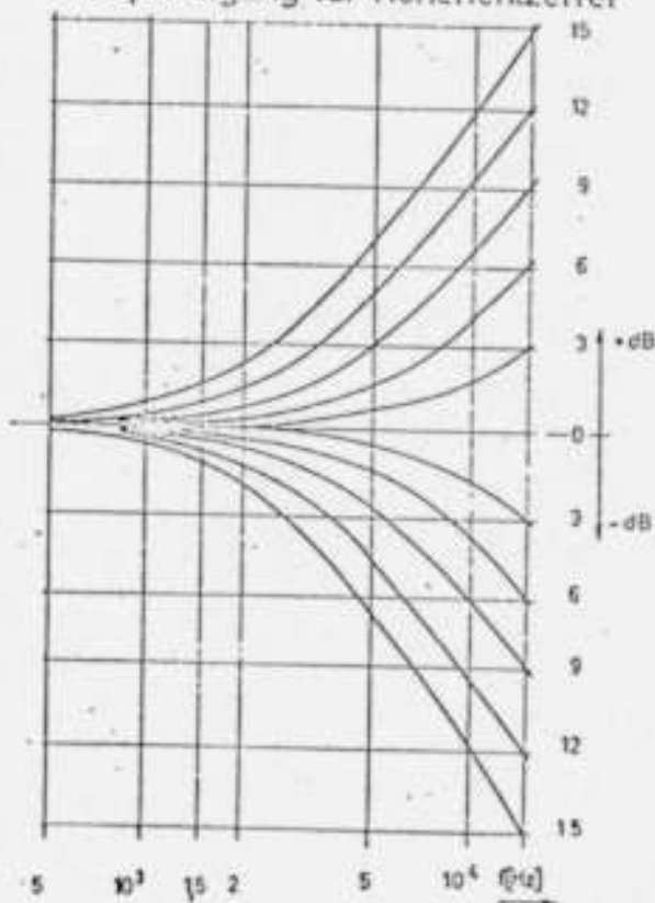
Frequenzgang für Höhenentzerrer
