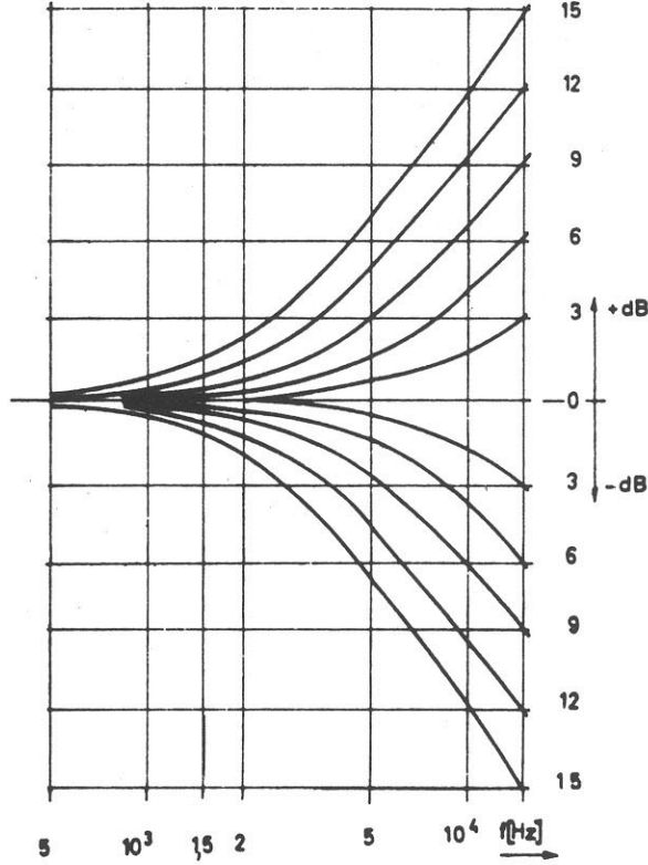
Frequenzgang für Höhenentzerrer
