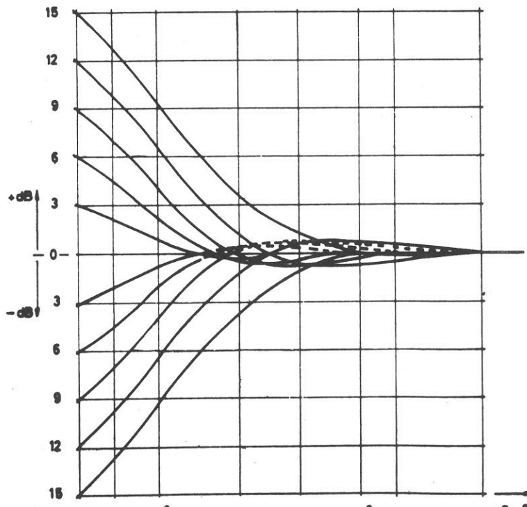
Frequenzgang für Tiefenentzerrer
