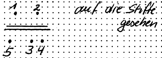
Anschlußschema / Skizze
