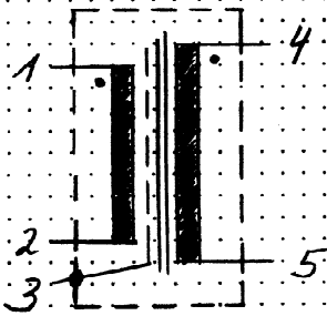
Schaltbild
